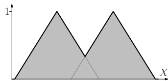
t -Konorm L_{\max}
