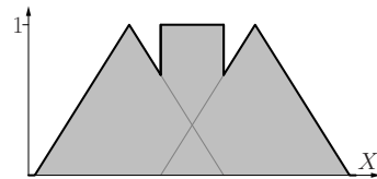
t -Konorm L_{-1}
