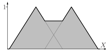
t -Konorm L_{\text{Luka}}
