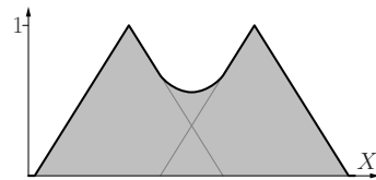
t -Konorm L_{\text{sum}}
