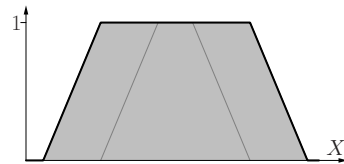
Fuzzy-Vereinigung
