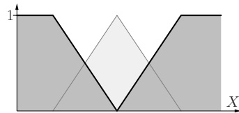
Fuzzy-Komplement
