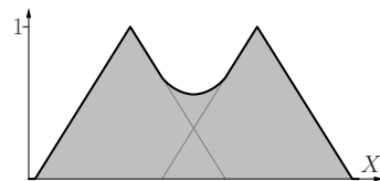
t -Konorm L_{\text{sum}}
