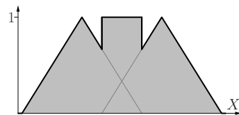
t -Konorm L_{-1}
