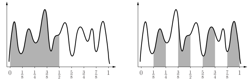
Schema 0**...*
