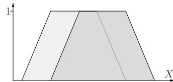
zwei Fuzzy-Mengen
